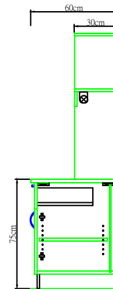
D-3 書桌, 書櫃, 抽櫃剖面圖
