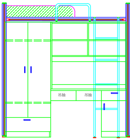
鋁合金床和全套家具立面圖
