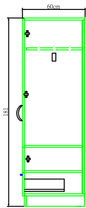
D-1 衣櫃剖面圖
