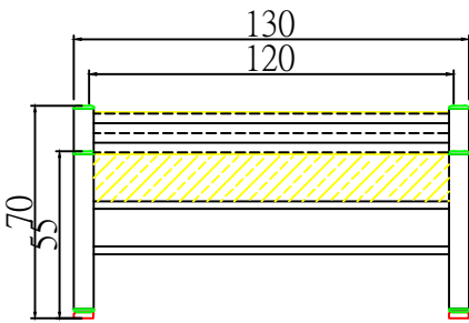
4尺單人床正面圖
